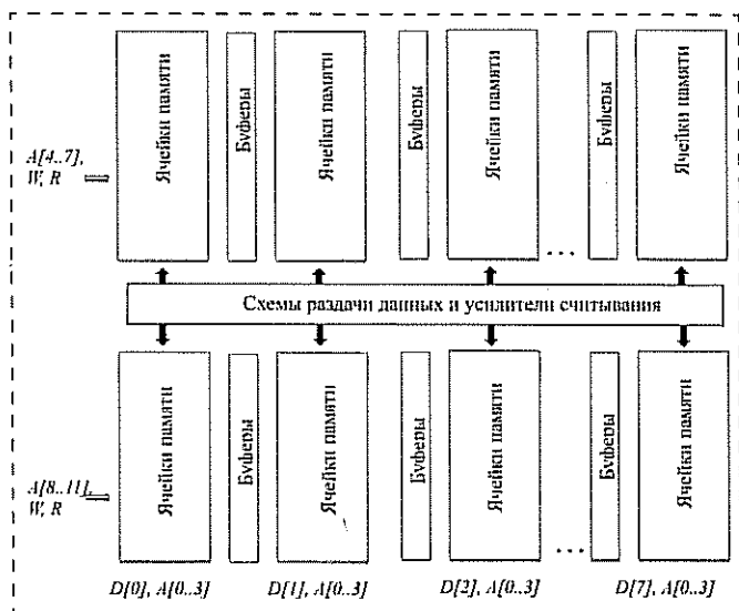
Пример организации матрицы ячеек для ОЗУ 4К×8: A[0..11] — адресная шина, W — команда записи, R — команда чтения, D[0..7] — шина данных
